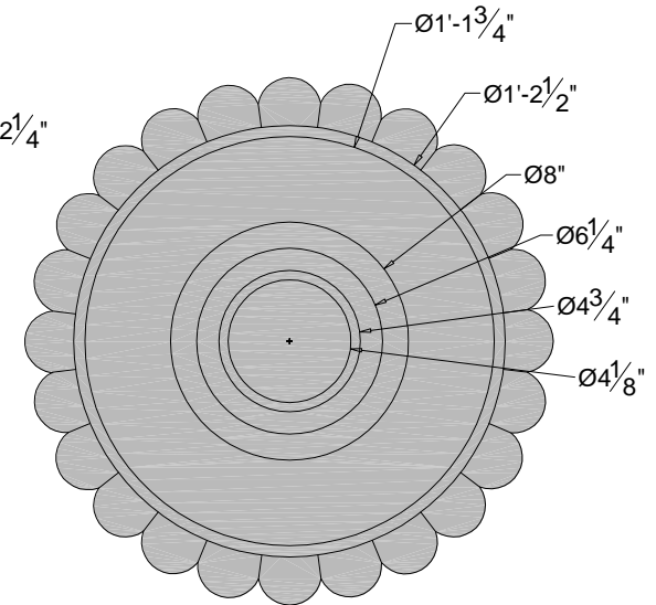
Bottom Elevation
