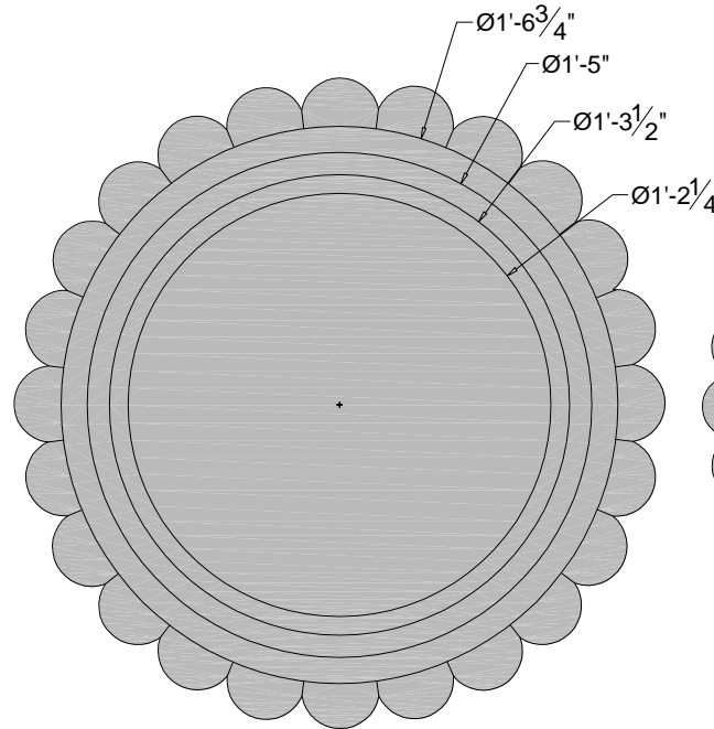
Top Elevation
