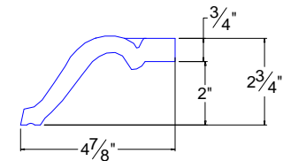
End Elevation
